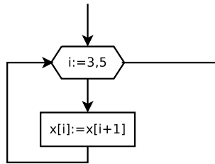
Рис. 5.25. Алгоритм удаления 3-го элемента из массива
