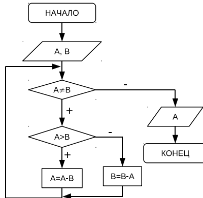
Рис. 3.28. Алгоритм поиска наибольшего общего делителя двух чисел
