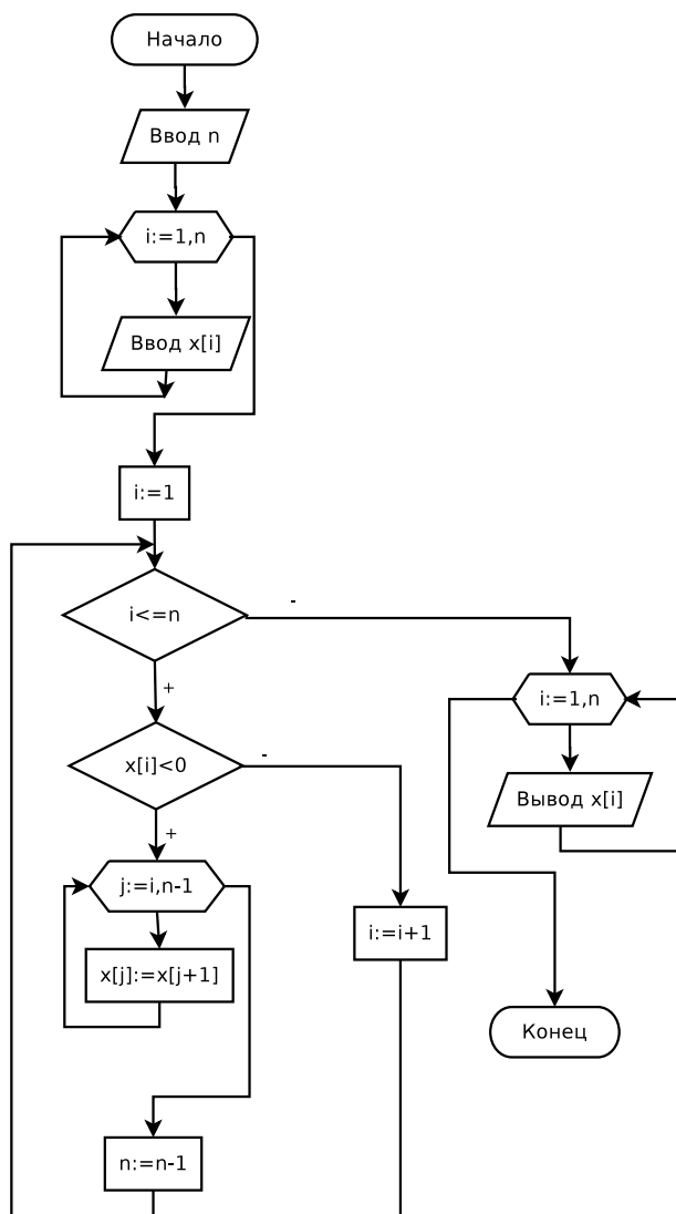
Рис. 5.28. Блок-схема решения задачи 5.1
