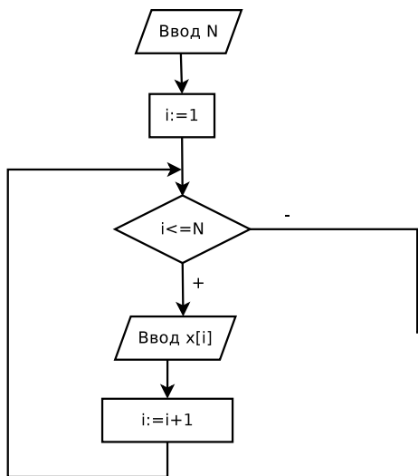
Рис. 5.3. Алгоритм ввода массива X с использованием цикла с предусловием
