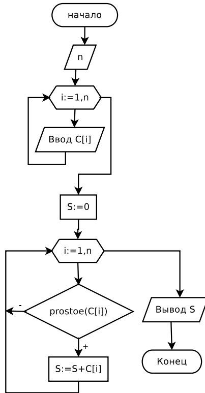
Рис. 5.38. Блок-схема решения задачи 5.7
