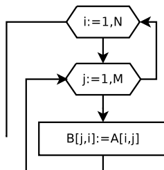
Рис. 6.6. Блок-схема транспонирования матрицы A
