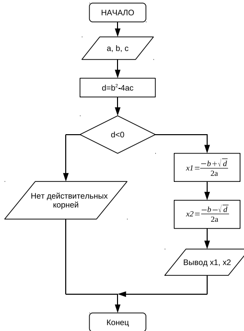
Рис. 3.14. Алгоритм решения квадратного уравнения
