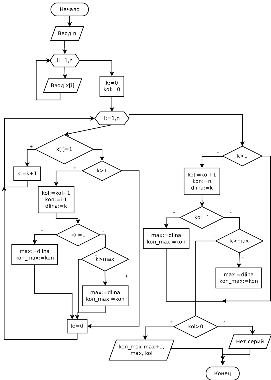
Рис. 5.41. Блок-схема решения задачи 5.9
