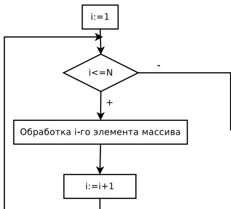
Рис. 5.1. Блок-схема обработки элементов массива с использованием цикла с предусловием
