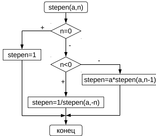
Рис. 4.10. Рекурсивный алгоритм вычисления степени числа
