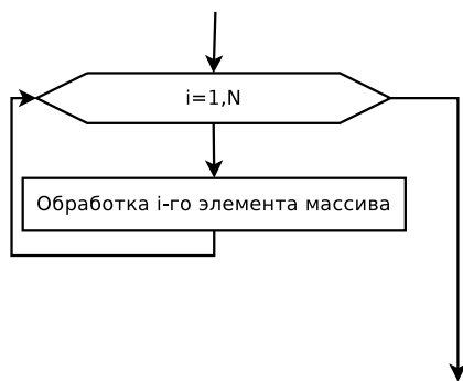
Рис. 5.2. Блок-схема обработки элементов массива с использованием цикла for
