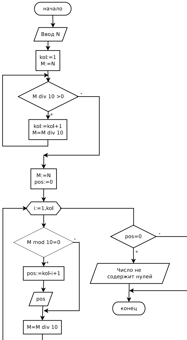
Рис. 3.36. Алгоритм решения задачи 3.17
