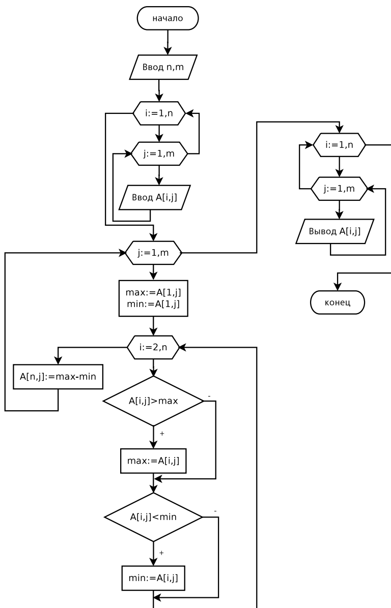
Рис. 6.20. Блок-схема алгоритма решения задачи 6.6
