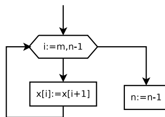
Рис. 5.27. Алгоритм удаления m -го элемента из массива из n элементов
