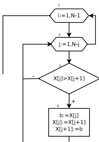
Рис. 5.22. Алгоритм упорядочения по возрастанию методом «пузырька»
