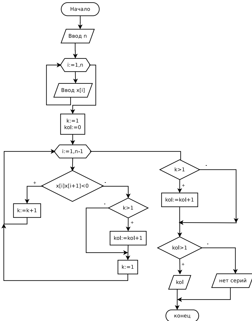
Рис. 5.40. Блок-схема решения задачи 5.8
