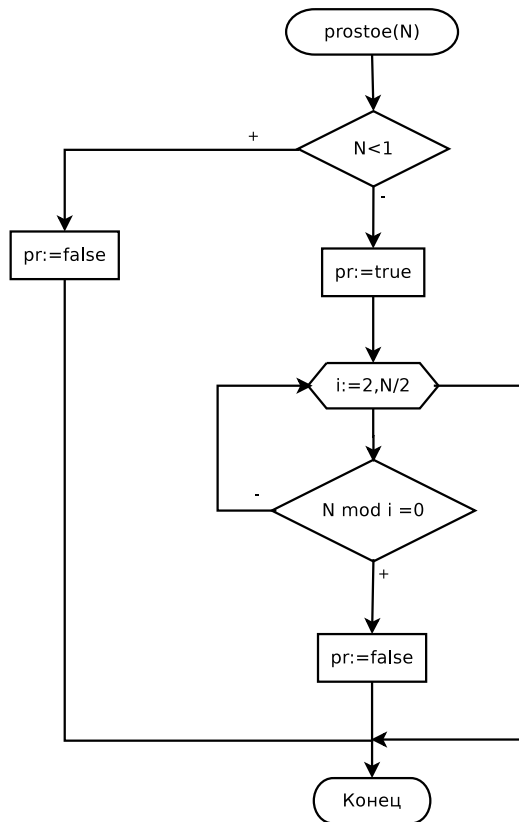
Рис. 5.37. Блок-схема функции prostoe
