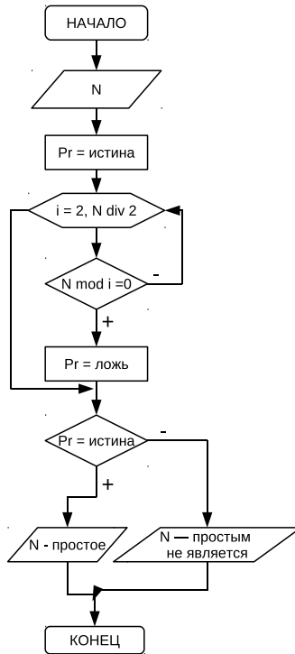
Рис. 3.33. Алгоритм определения простого числа
