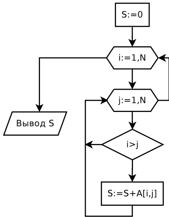
Рис. 6.14. Блок-схема задачи 6.3 (алгоритм 1)
