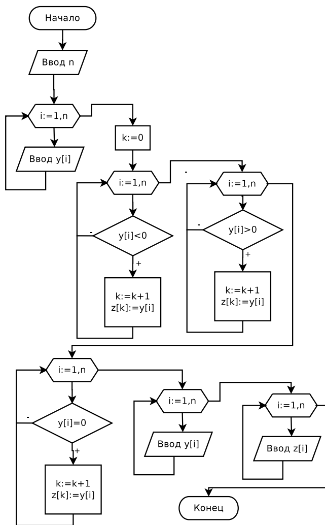
Рис. 5.34. Блок-схема решения задачи 5.4
