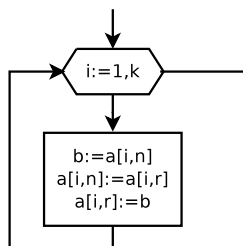
Рис. 6.23. Блок-схема алгоритма решения задачи 6.7
