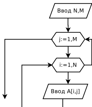
Рис. 6.3. Блок-схема ввода элементов матрицы
