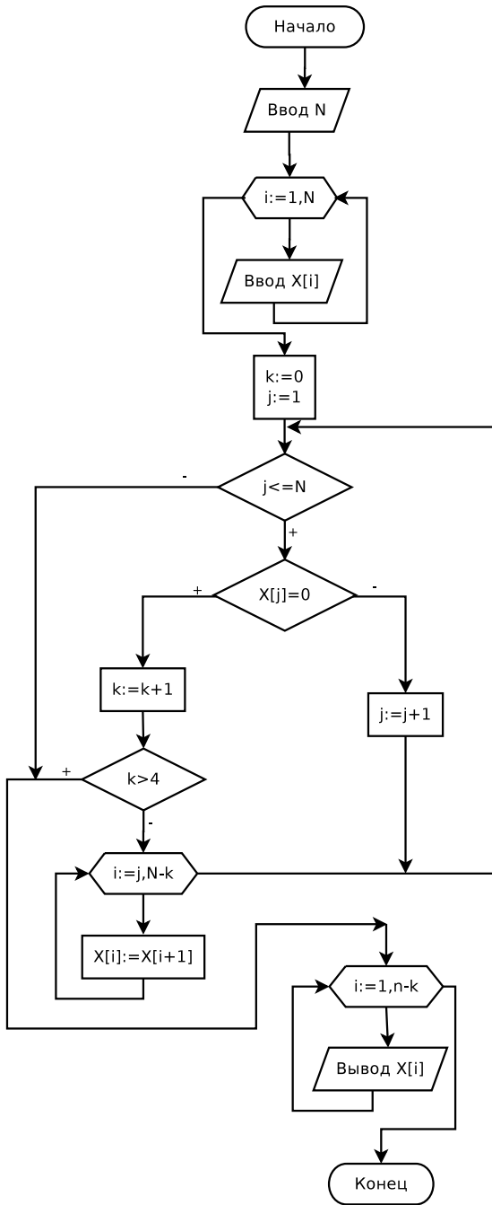
Рис. 5.36. Алгоритм решения задачи 5.6
