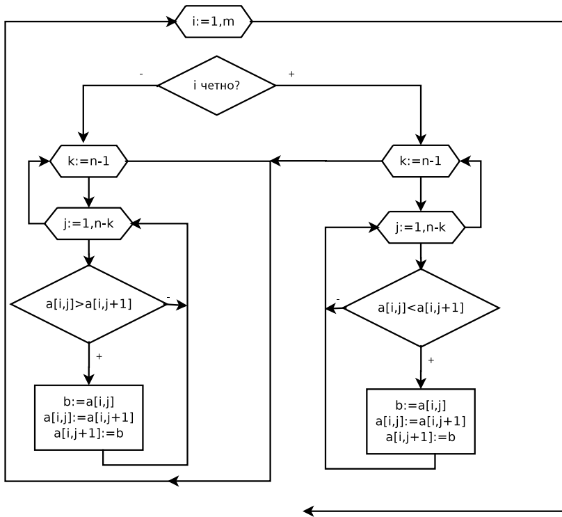
Рис. 6.25. Блок-схема алгоритма решения задачи 6.8
