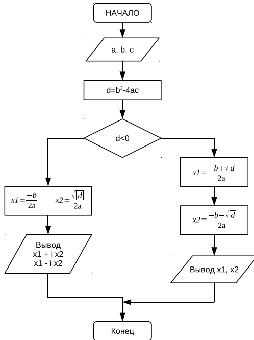
Рис. 3.15. Алгоритм решения задачи 3.4
