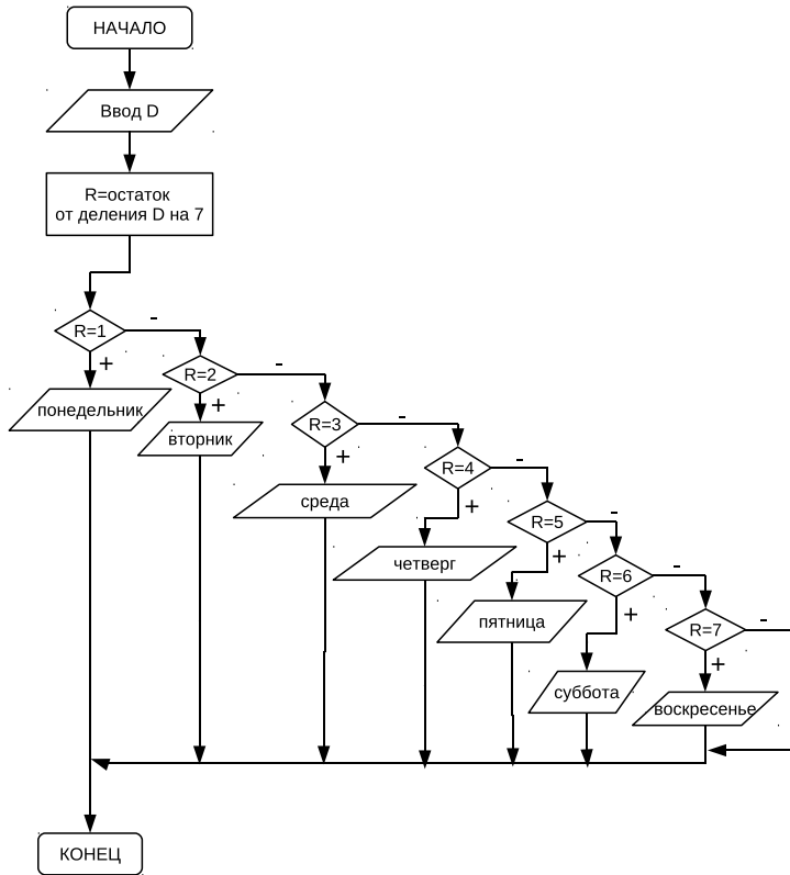
Рис. 3.18. Алгоритм решения задачи 3.7
