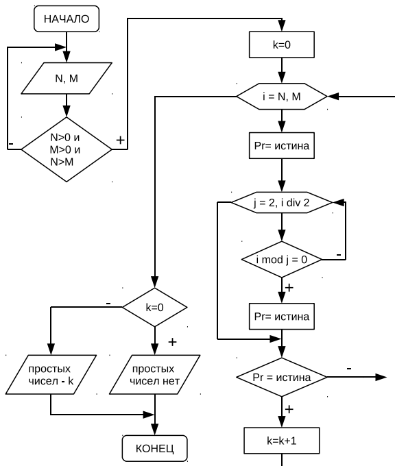
Рис. 3.34. Алгоритм определения простых чисел в заданном интервале
