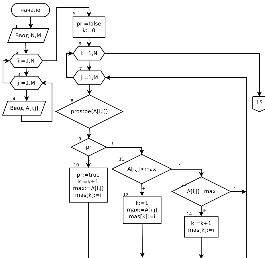
Рис. 6.33. Блок-схема решения задачи 6.11 (начало)
