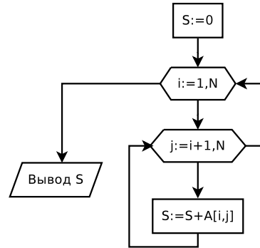
Рис. 6.15. Блок-схема задачи 6.3 (алгоритм 2)
