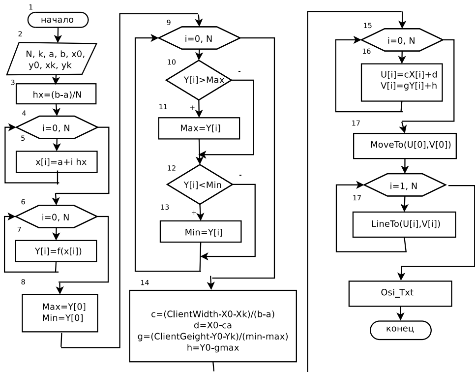
Рис. 10.3. Блок-схема алгоритма построения графика функции
