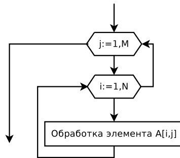
Рис. 6.2. Алгоритм обработки матрицы по столбцам
