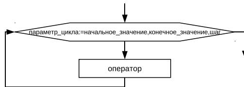
Рис. 3.27. Представление цикла for...do с помощью блок-схемы
