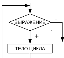
Рис. 3.24. Алгоритм циклической структуры с предусловием
