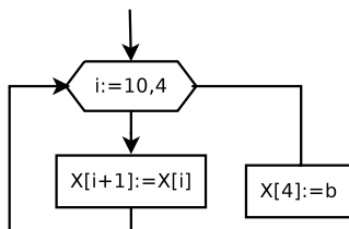
Рис. 5.30. Вставка числа b между третьим и четвёртым элементов массива X
