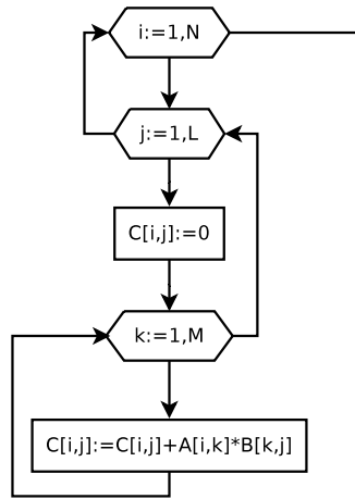
Рис. 6.29. Блок-схема умножения двух матриц
