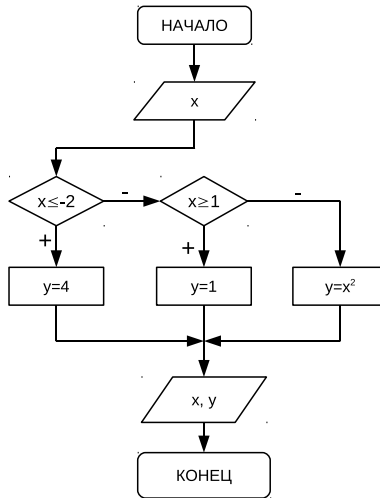
Рис. 3.11. Блок-схема алгоритма решения задачи 3.1
