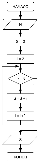
Рис. 3.31. Алгоритм вычисления суммы чётных натуральных чисел
