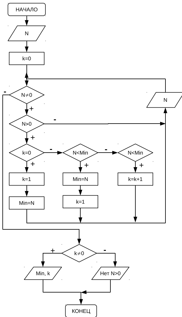
Рис. 3.43. Алгоритм поиска минимального положительного числа в последовательности
