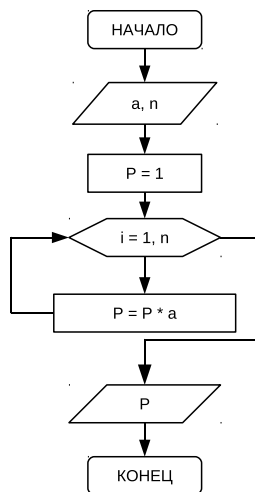
Рис. 3.30. Алгоритм возведения вещественного числа в целую степень
