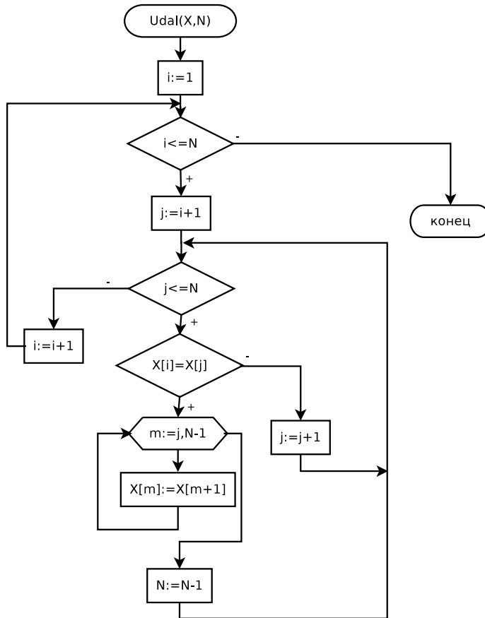
Рис. 6.31. Блок-схема процедуры Udal
