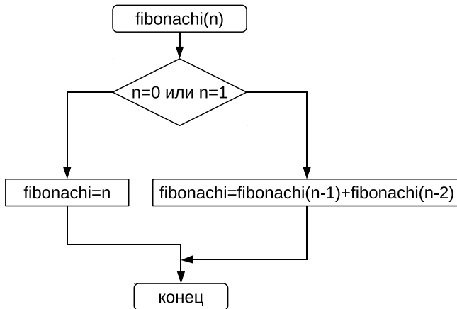
Рис. 4.11. Рекурсивный алгоритм вычисления числа Фибоначчи
