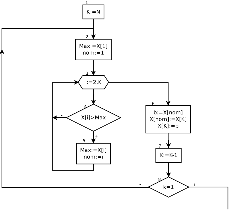
Рис. 5.24. Сортировка массива по возрастанию выбором наибольшего элемента
