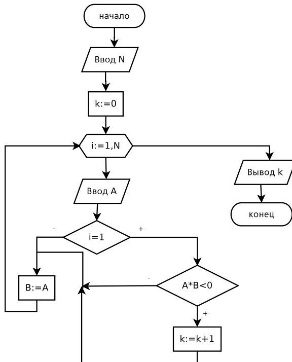
Рис. 3.44. Алгоритм к задаче 3.20
