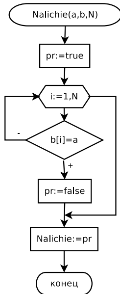
Рис. 6.32. Блок-схема функции Nalichie
