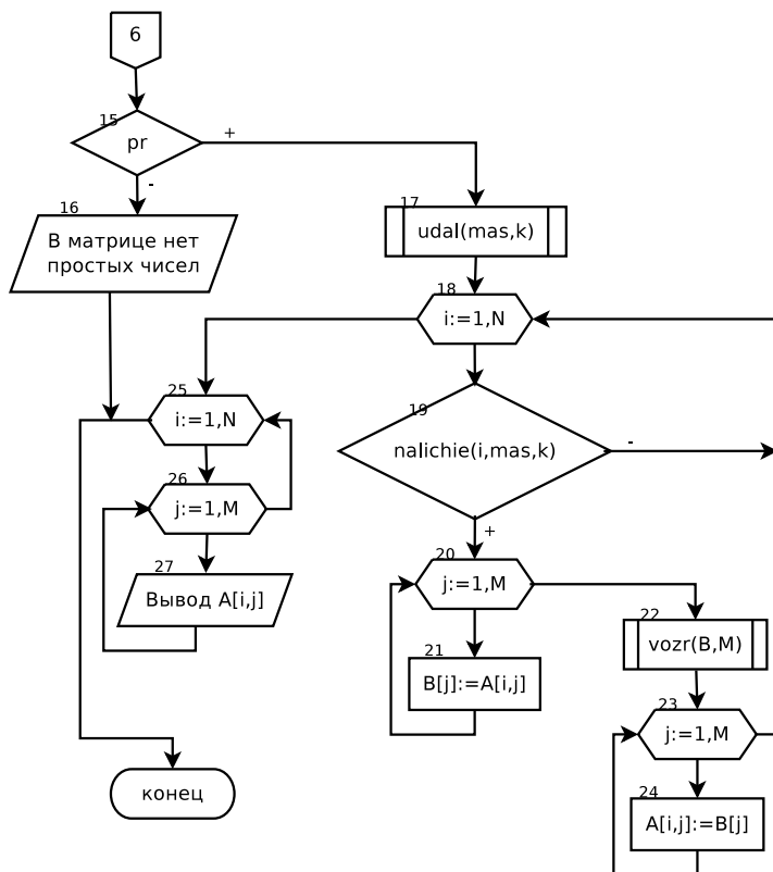
Рис. 6.34. Блок-схема решение задачи 6.11 (продолжение)
