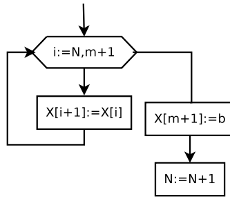
Рис. 5.31. Вставка числа b в массив X
