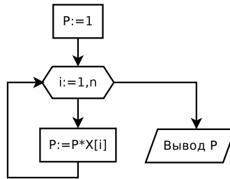
Рис. 5.20. Алгоритм нахождения произведения элементов массива
