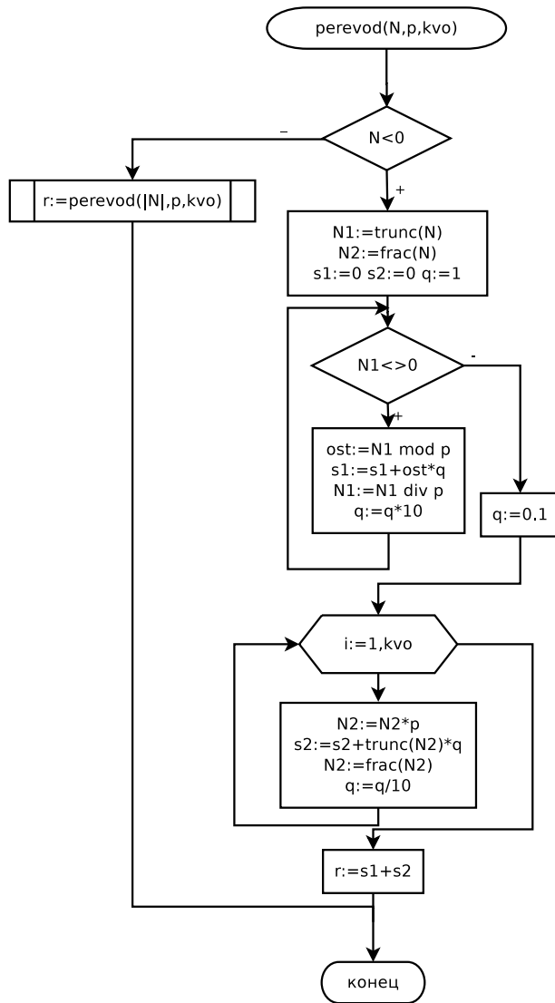
Рис. 5.42. Блок-схема функции перевода вещественного числа в p -ричную систему счисления
