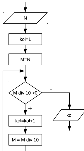
Рис. 3.35. Алгоритм определения количества цифр в числе
