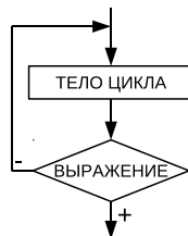
Рис. 3.25. Алгоритм циклической структуры с постусловием
