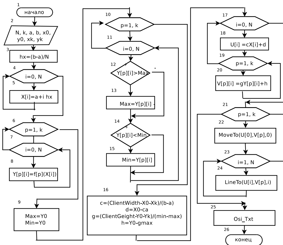
Рис. 10.4. Блок-схема алгоритма построения графиков нескольких функций
