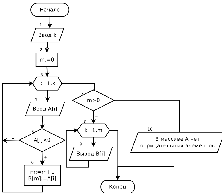
Рис. 5.33. Блок-схема формирования массива B из отрицательных элементов массива A
