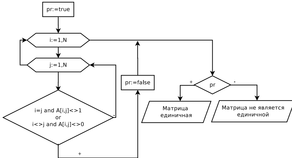
Рис. 6.19. Блок-схема алгоритма решения задачи 6.5
