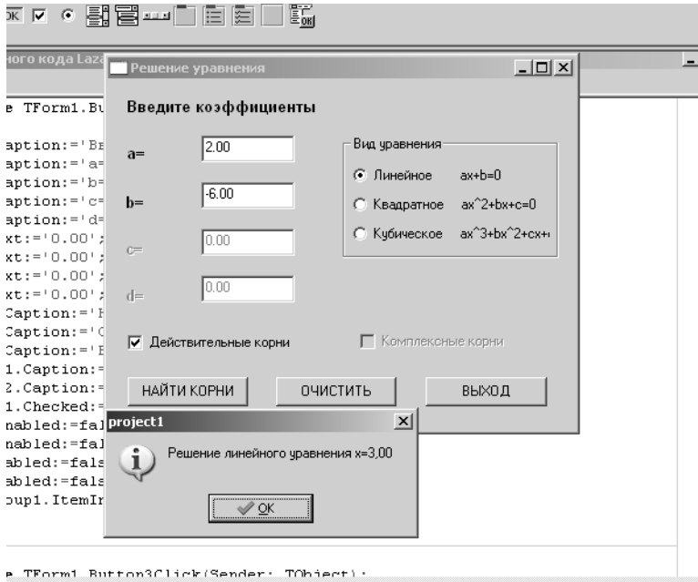
Рис. 4.6. Решение линейного уравнения
