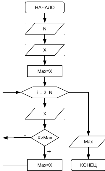
Рис. 3.38. Алгоритм поиска наибольшего числа в последовательности
