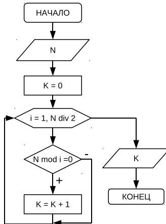
Рис. 3.32. Алгоритм подсчёта делителей натурального числа
