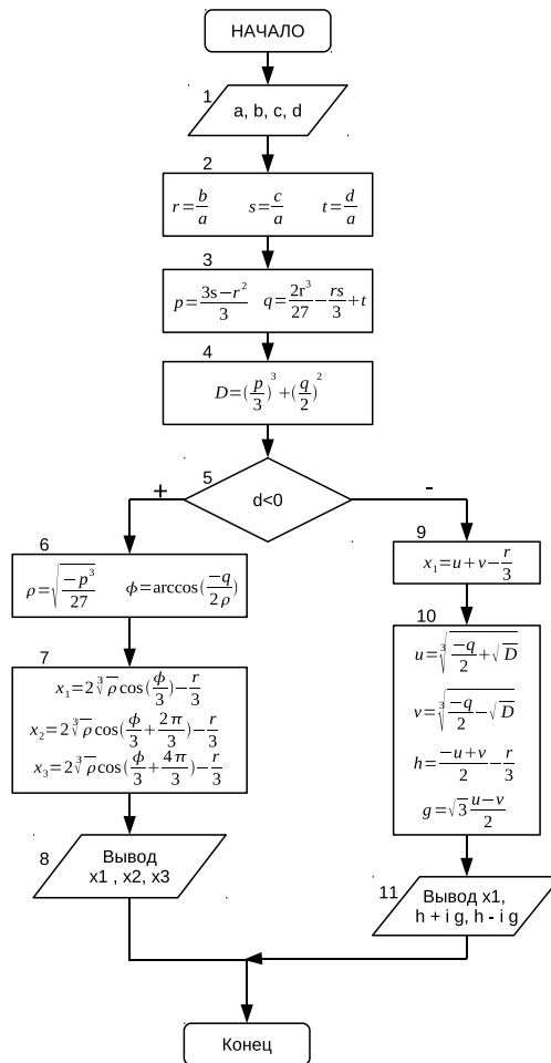
Рис. 3.16. Алгоритм решения кубического уравнения
