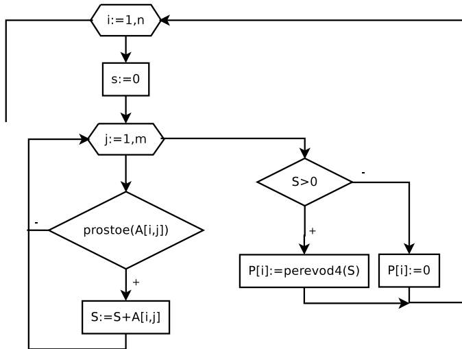
Рис. 6.27. Блок-схема алгоритма решения задачи 6.9
