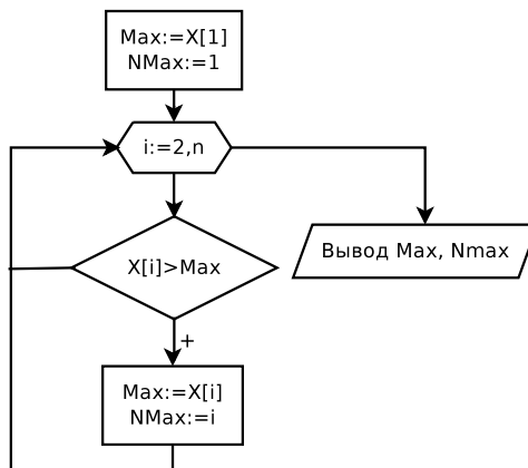
Рис. 5.21. Алгоритм поиска максимального элемента массива и его номера
