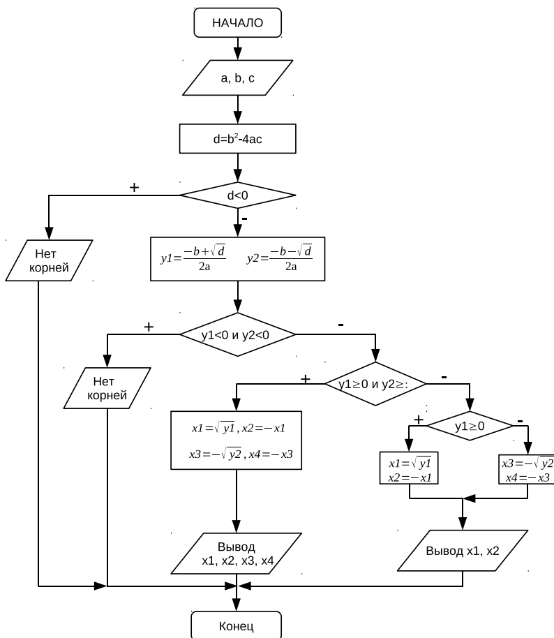
Рис. 3.17. Алгоритм решения биквадратного уравнения
