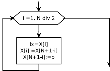
Рис. 5.35. Фрагмент блок-схемы к задаче 5.5
