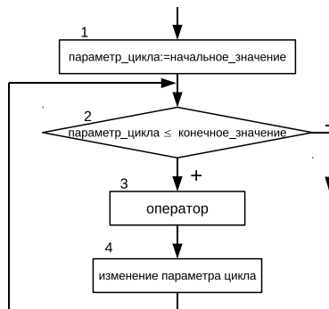
Рис. 3.26. Алгоритм работы цикла for..do
