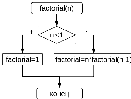
Рис. 4.9. Рекурсивный алгоритм вычисления факториала
